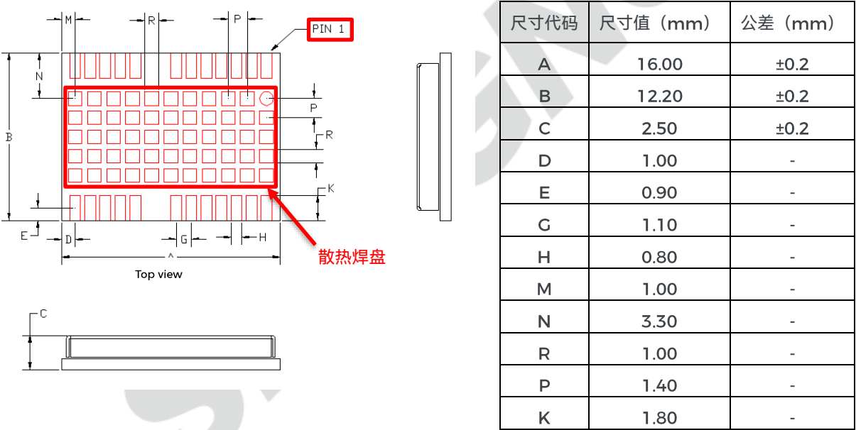
Figure 2. K901 机械图
